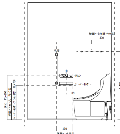
便器~手摺芯
