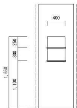
□ パターンJ H550×W400
