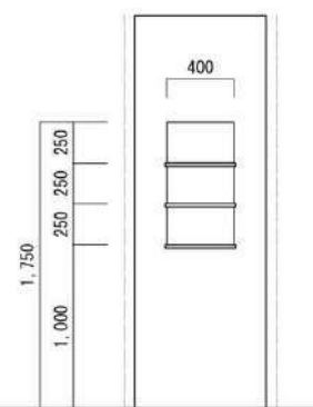
□ パターンL H750×W400
