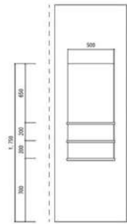
□ パターンD H1050×W500 (H650・H200・H200 台有に限る) ※リモコンニッチ可能
